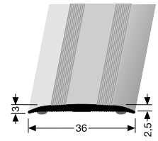
PF 440 SK selbstklebend self-adhesive auto-adhésif
