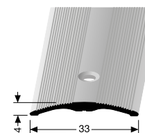
PF 231 mittig versenkt gebohrt centrally countersunk drilled à percement noyé central
