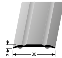
PF 439 SK selbstklebend self-adhesive auto-adhésif
