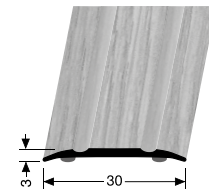
PF 439 H/SK mit Holzdekor, selbstklebend with wood decor, self-adhesive avec décor bois, auto-adhésif
