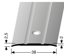
PF 438 mittig versenkt gebohrt centrally countersunk drilled à percement noyé central
