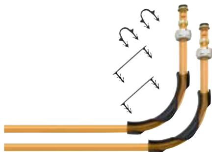
Elosztó-csatlakozó készlet komponensei 16 mm átmérőjű fűtőcsővekhez
