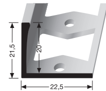
PF 313 G \varnothing 20 mm geschlossen gestanz perforated base estampé fermé
