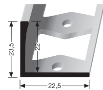
PF 309 G \varnothing 22 mm geschlossen gestanz perforated base estampé fermé
