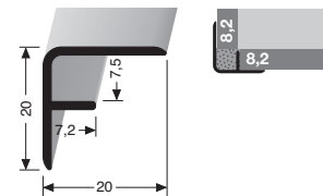
PF 165 U \updownarrow 8,2 mm Kombi Innen- /Außenecke, ungebohrt Combi internal/external corner, undrilled Combi coin intérieur/extérieur, non percé
