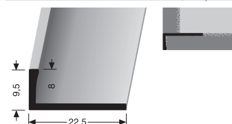
PF 303 U \updownarrow 8 mm Abschlussprofile, ungebohrt Border profile, undrilled Seuil d'arrêt, non percé
