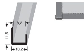
PF 178 U \updownarrow 8,2 mm Abschlussprofile, ungebohrt Border profile, undrilled Seuil d'arrêt, non percé
