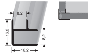
PF 164 U \updownarrow 8,2 mm Kombi Innen- /Außenecke, ungebohrt Combi internal/external corner, undrilled Combi coin intérieur/extérieur, non percé
