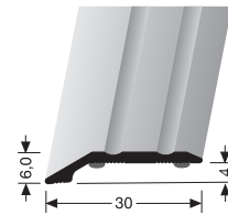
PF 240 SK selbstklebend self-adhesive auto-adhésif
