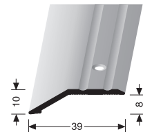
PF 244 versenkt gebohrt countersunk drilled à percement noyé
